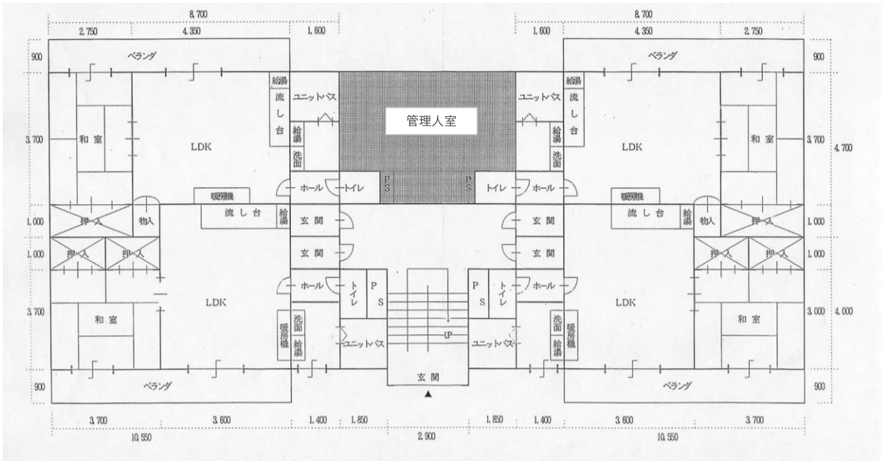
1階平面図(1LDK)
