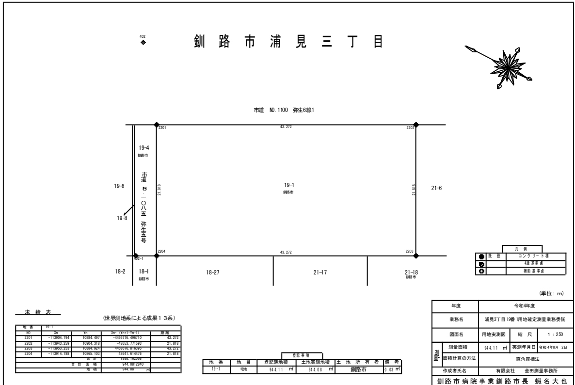
実測平面図
