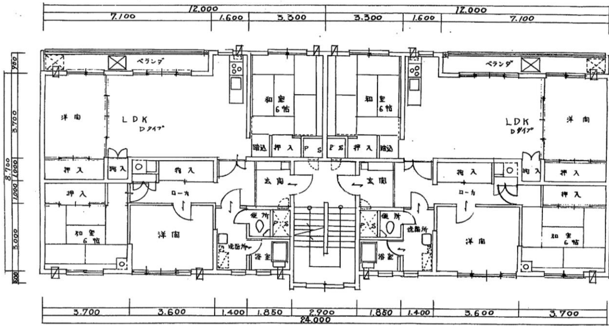
2～3階平面図(4LDK)
