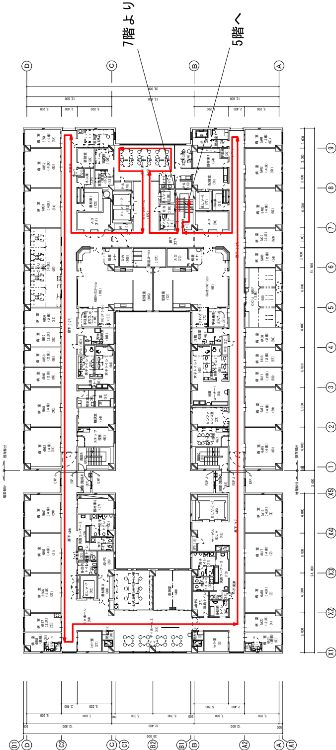
市立釧路総合病院 6階平面図
