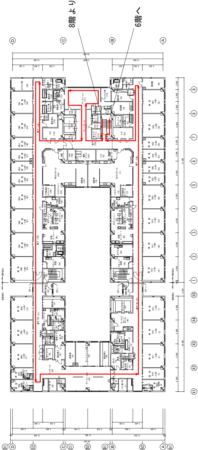
市立釧路総合病院 7階平面図
